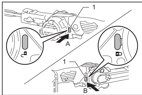
► 1. Interrupteur de sécurité
