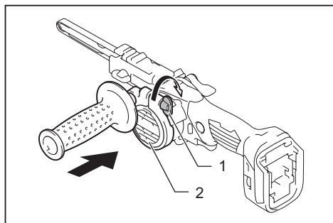
► 1. Tornillo de mariposa 2. Alojamiento del motor
