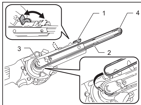
► 1. Palanca de leva 2. Banda abrasiva 3. Polea trasera 4. Polea delantera
