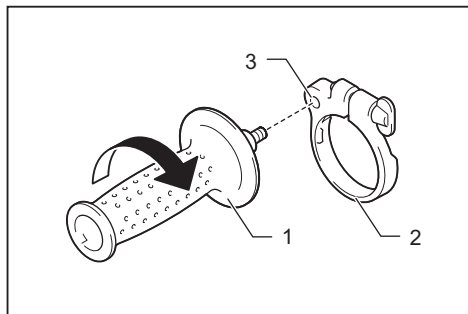
► 1. Empuñadura 2. Base de la empuñadura 3. Tuerca de sujeción
